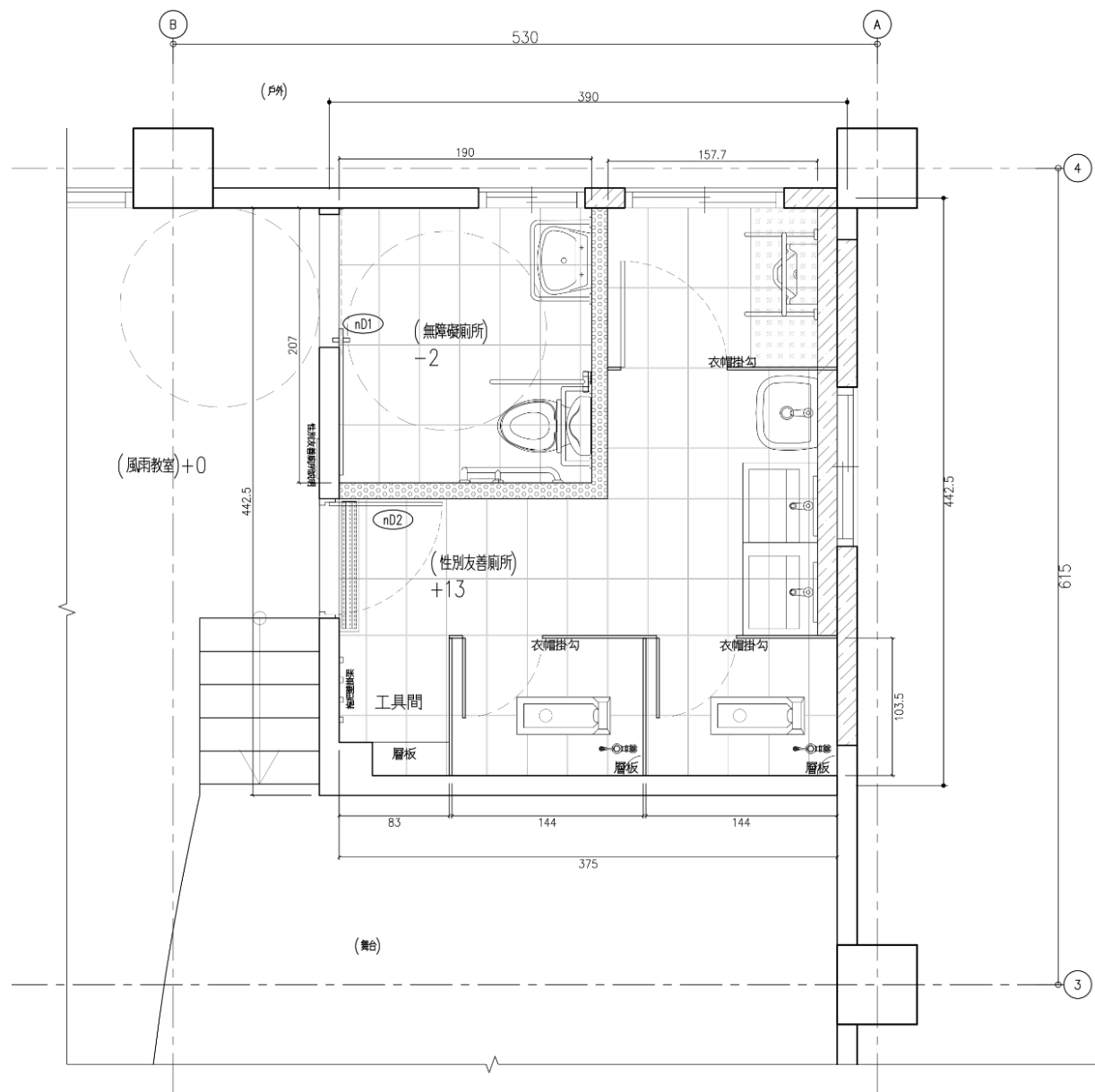
性別友善廁所設計平面圖
